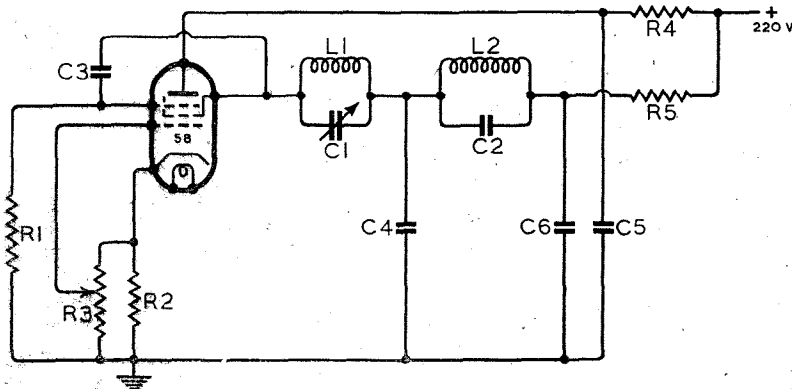
Fig. 1. Original Transitron oscillator circuit. Values of components: R_1 , 100,000 \Omega ; R_2 , 2,000 \Omega ; R_3 , 0.5M \Omega ; R_4 , 7,500 \Omega ; R_5 , 25,000 \Omega ; C_1 , 0.0005 \mu F; C_2 , 0.03 \mu F; C_3 , 0.01 \mu F; C_4 , 10 \mu F; C_5 , 1 \mu F; C_6 , 1 \mu F.
